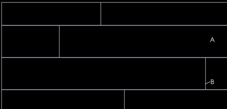
DECK BLOCK Option 1: 76,2 x 914,4 mm Option 2: 114,3 x 914,4 mm Stripping optional: 3,2 x 914,4 mm
